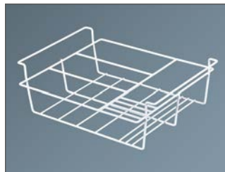
SCOOP BASKET: KURVSCOOPF3+1 W X H: 442 X 123 MM
